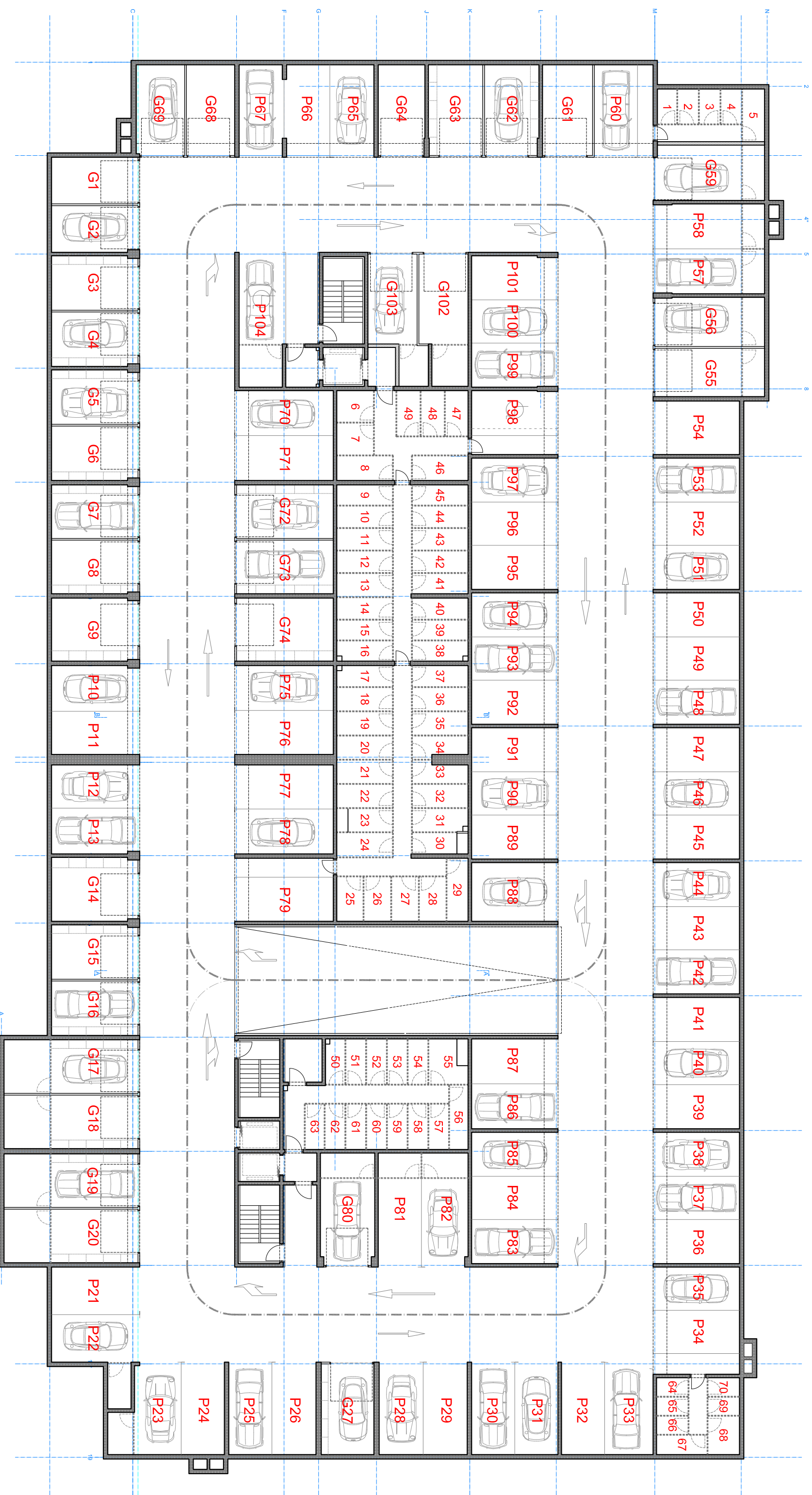
TLOCRT PODRUMA -1
